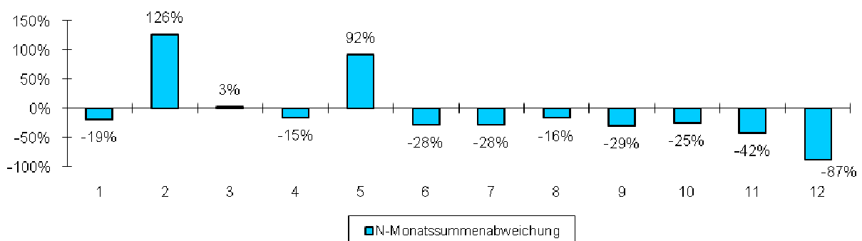
Abb.1: Monatlicher Niederschlag 2018 im Vergleich zum langjährigen Mittel in Klagenfurt (Quelle: Hydrographischer Landesdienst)
